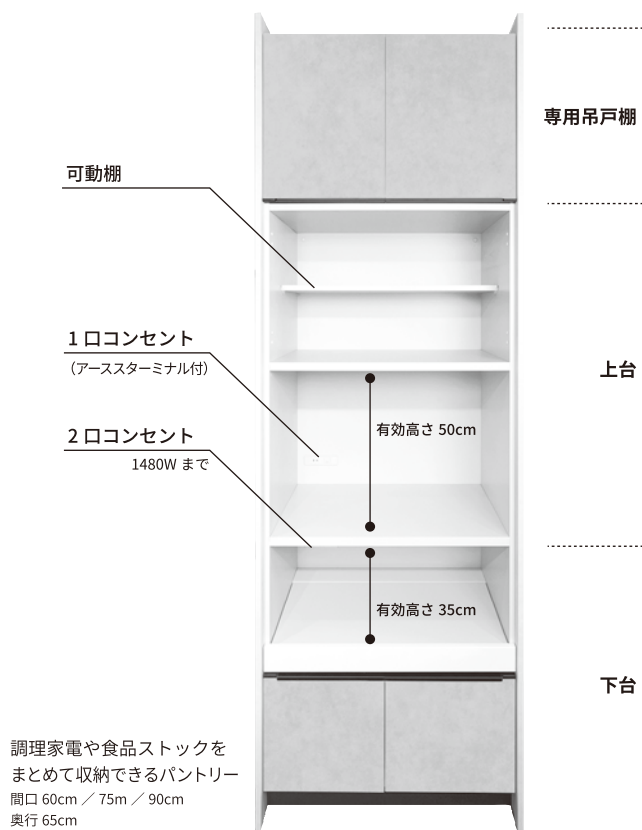
専用吊戸棚 (開き扉)
