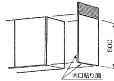
吊戸棚
