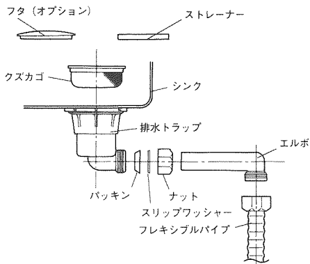
排水トラップセット図
